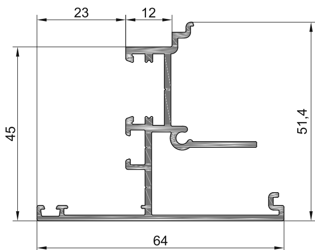
Штульповый профиль
