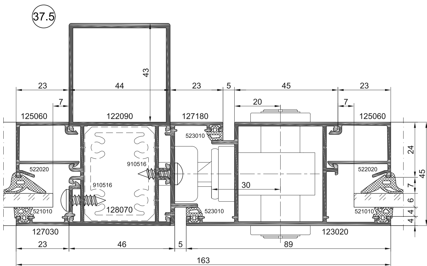
Однопольная дверь Открытие наружу 43
