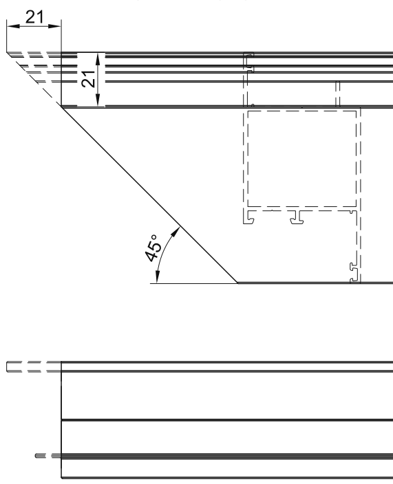
Обработка профиля 123030
