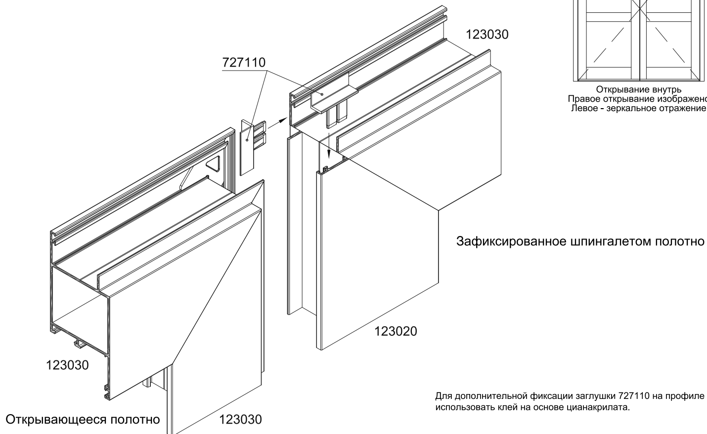
Обработка профиля 123020
