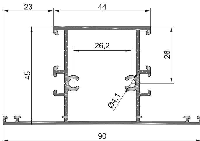
Импостный профиль 44 мм под саморезы
