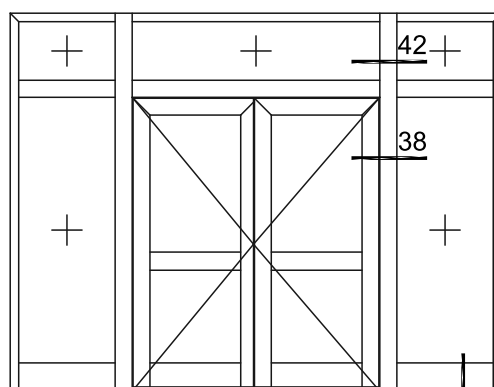
Двупольная дверь Открытие наружу 43
