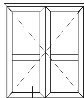
Двупольная дверь со ступом Открытие внутрь
