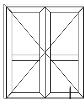
22 Двупольная дверь со штульпом Открытие наружу
