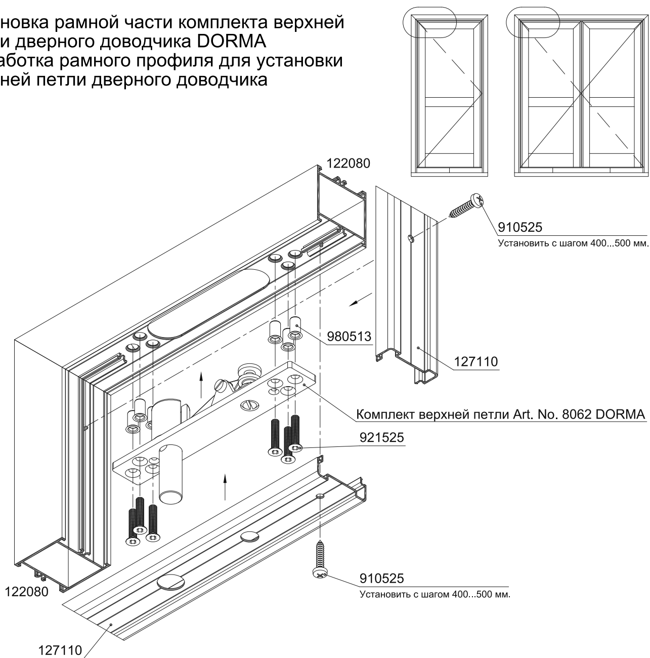
Обработка рамного профиля 122080
