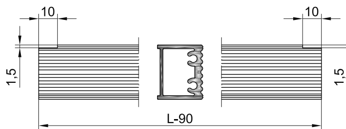
Обработка профиля порога 127171
