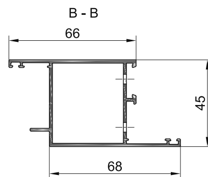
Б - Б
