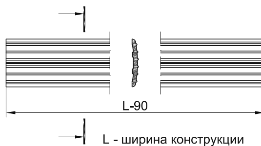
Обработка профиля порога 127160
