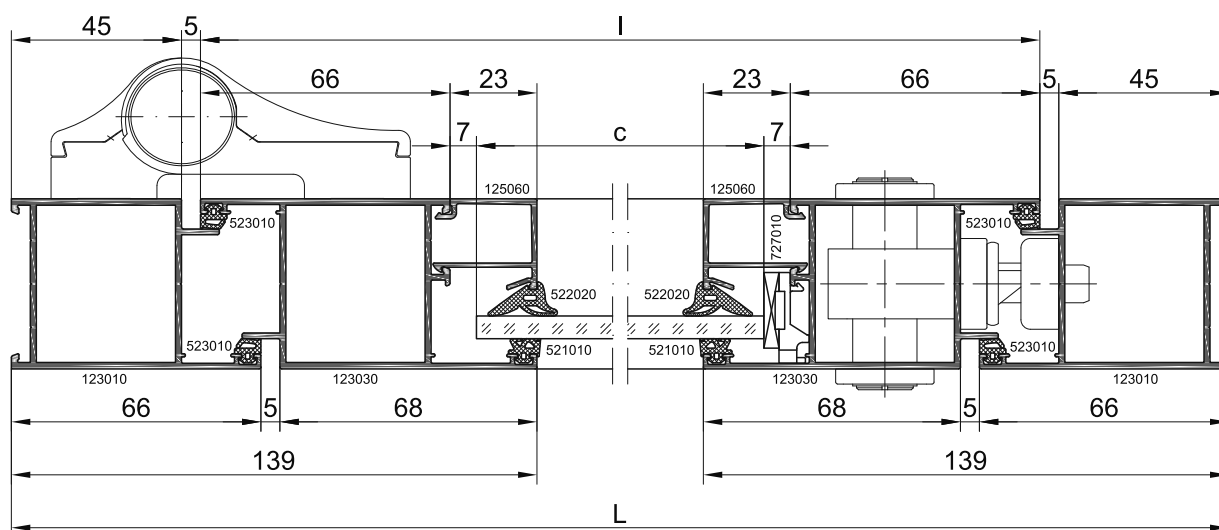
A - A
