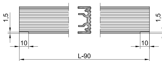
L - ширина конструкции
