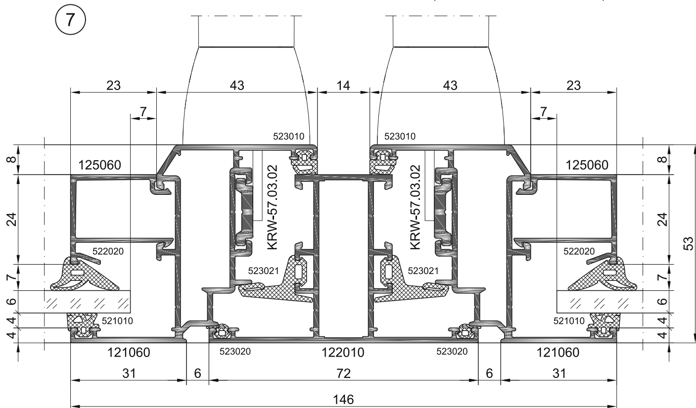
Комбинированное окно
