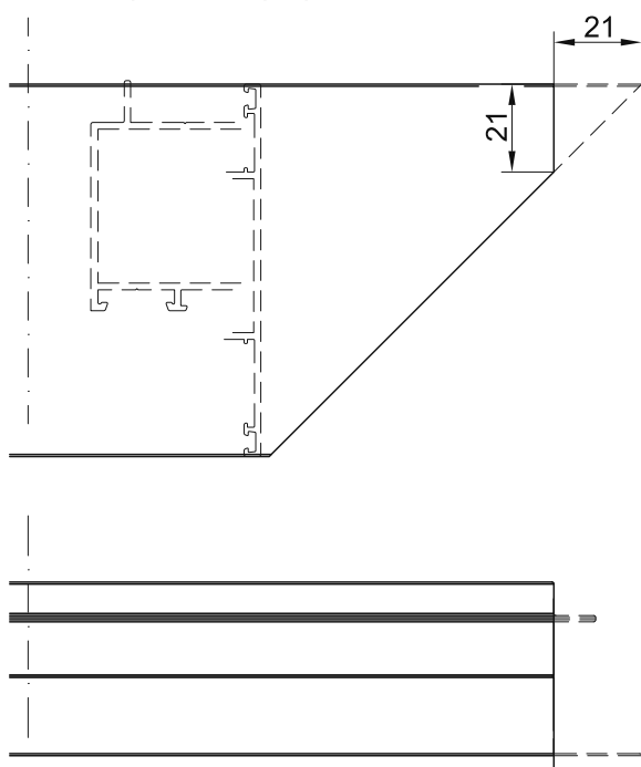
Обработка профиля 123020
