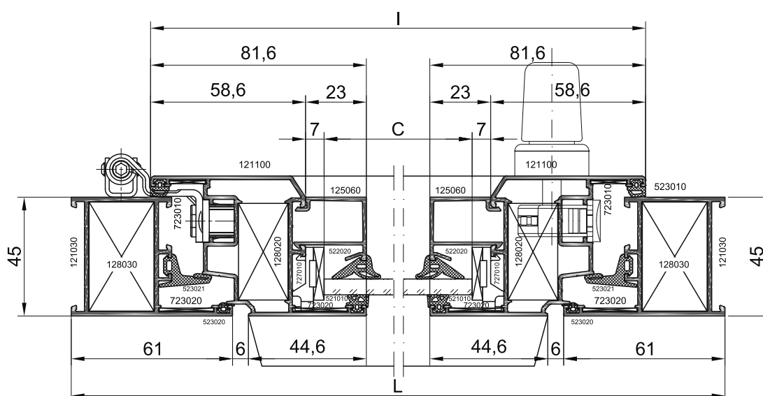
A - A
