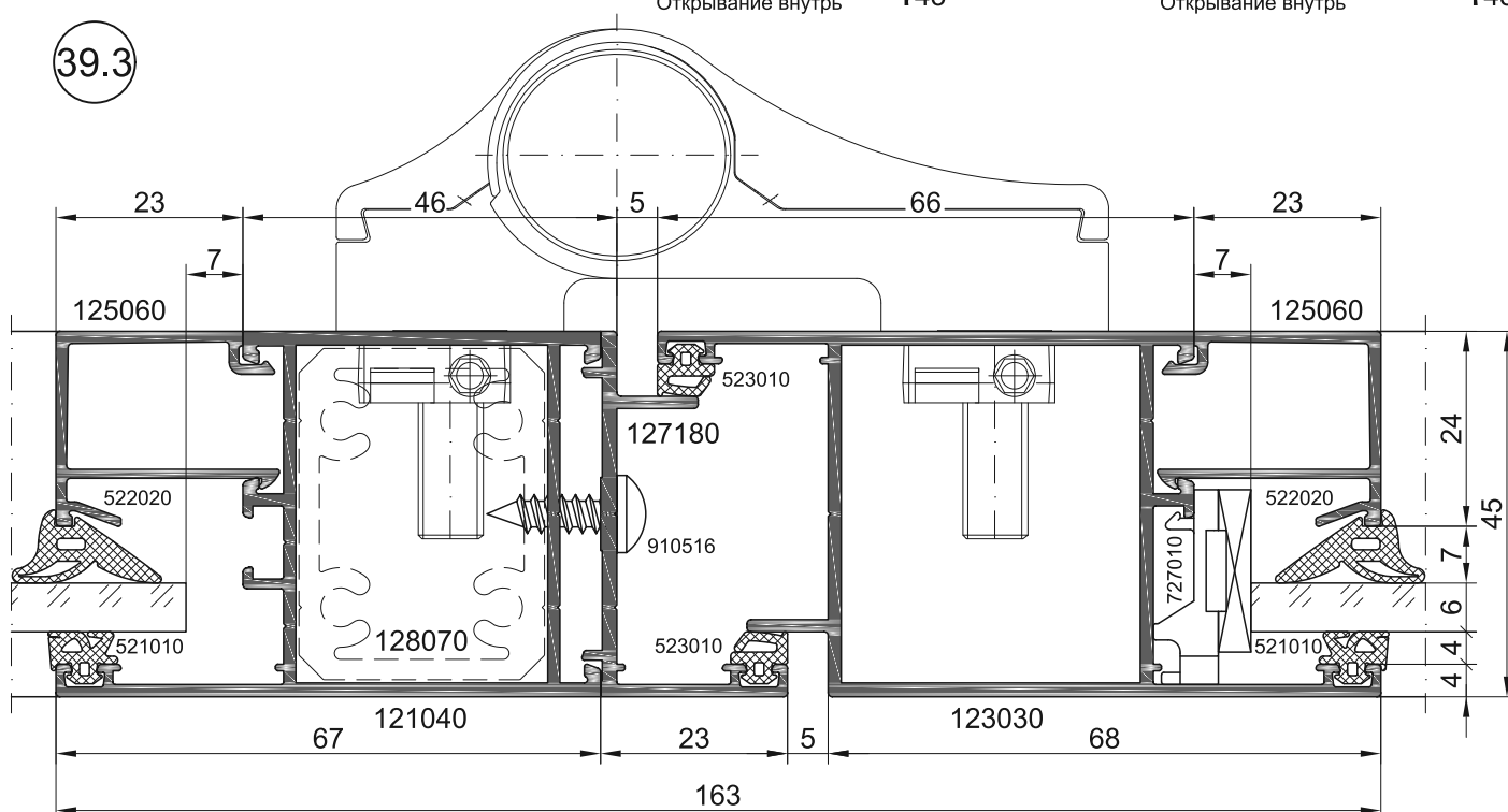
Однополюсная дверь Открытие внутрь
