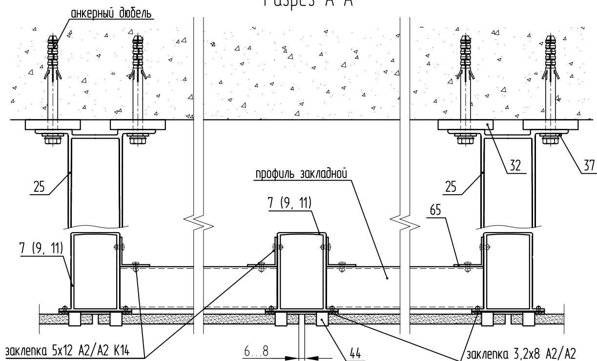
Разрез А-А
