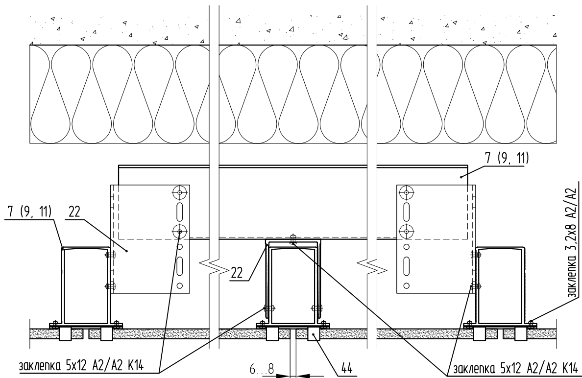
Разрез А-А
